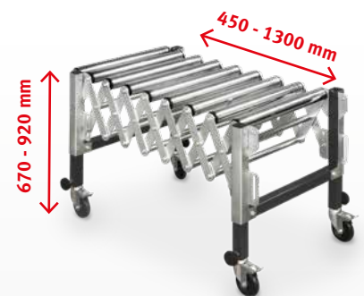
SRB 130 Scherenrollenbahn Höhe einstellbar, Rollenlänge 480 mm
